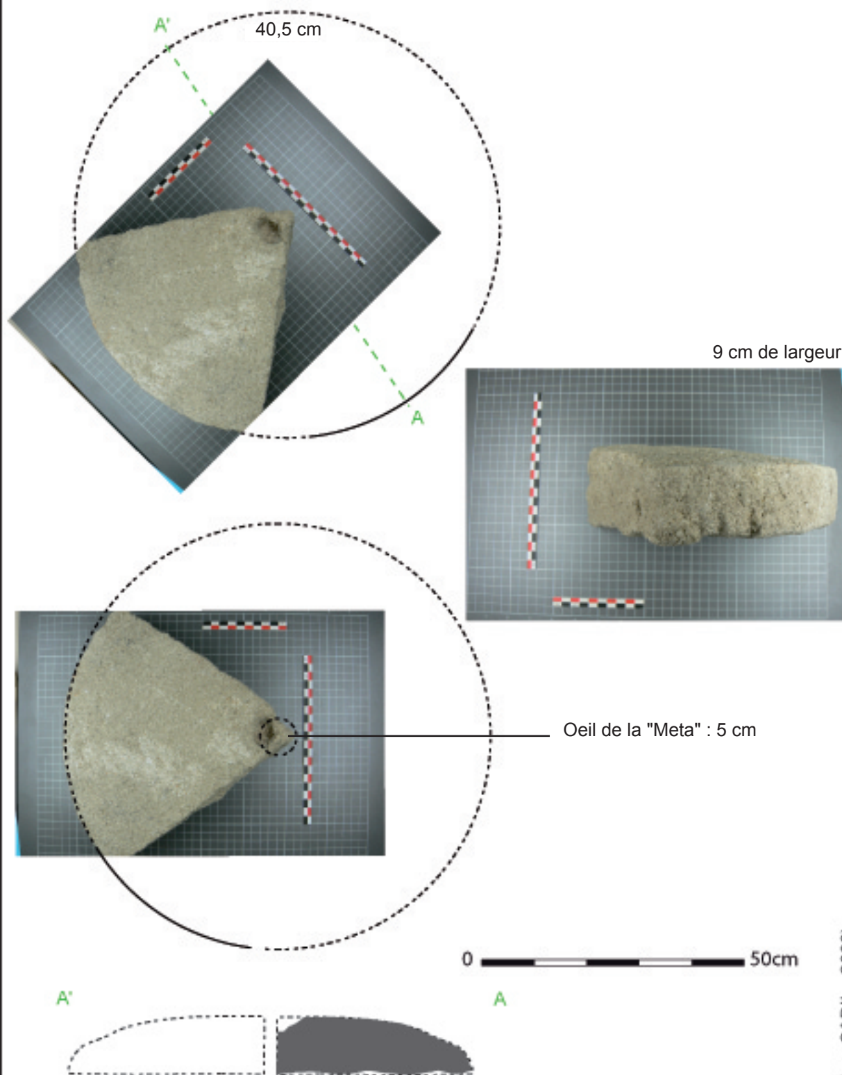
Fragment de meule (partie rotative), face supérieure et coupe US 3000 (décapage) Poids : 4730 g "Le Moulin d'Epigny". Ligueil (37)
