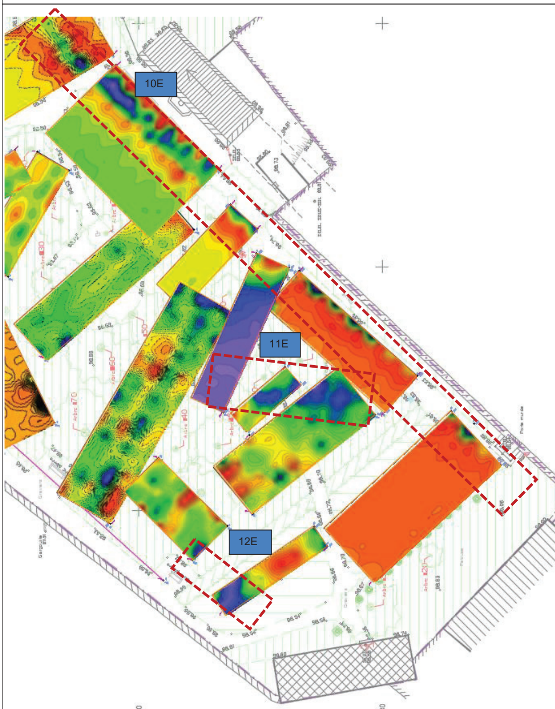
Figure 17 : mapping de la partie sud du site par méthode électromagnétique à induction
