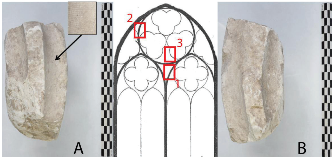
Fig. 22 : Faces des embrasures interne (A) - avec détail des traces de ripe - et externe (B) du lot 623 et restitution de la position du fragment sur un arc (1), un oculus (2) ou une forme polylobée (3) (M. Beigneux, CD37 et S. Bourocher).
