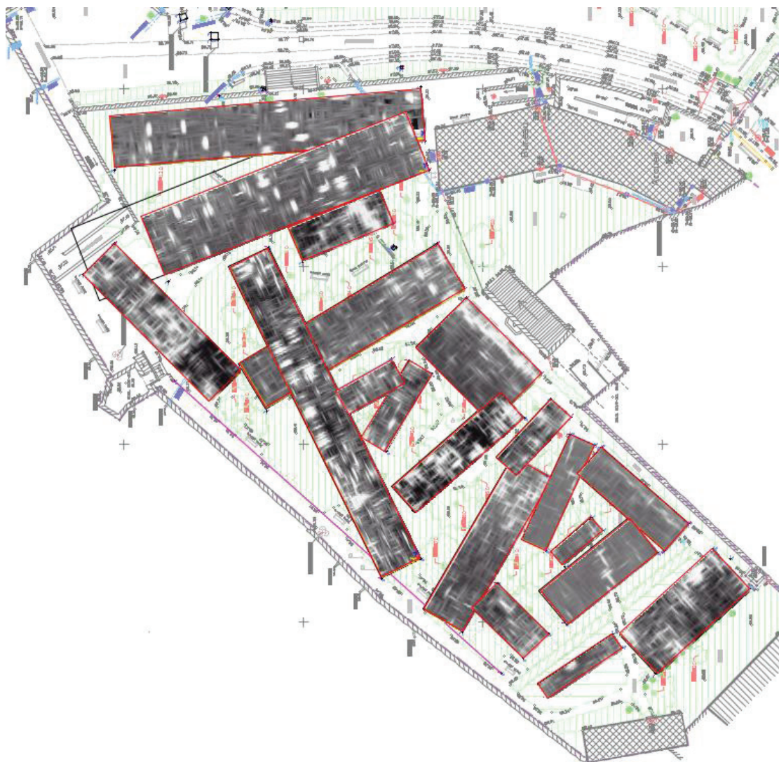
Figure 11 : mapping radar haute fréquence en z = 0.40 et 0.60 m
