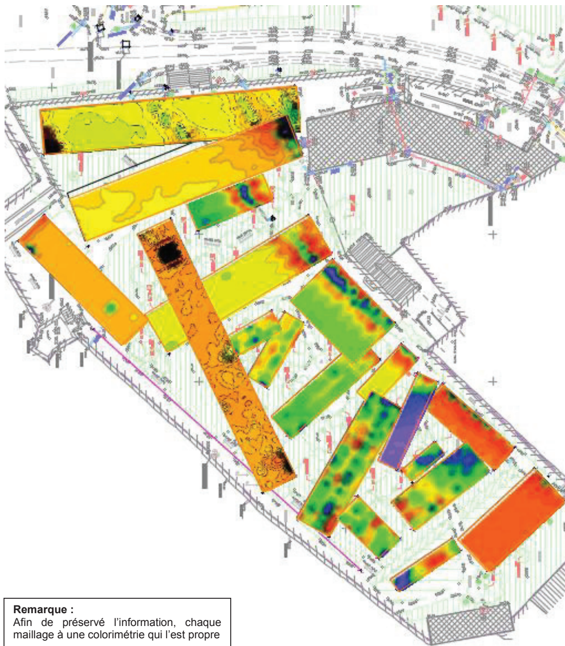
Figure 15 : mapping en z = 0.75 m de la méthode électromagnétique à induction
