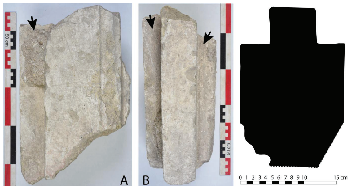
Fig. 28 : Face d'ébrasement (A), face interne (B) et profil du lot 629 avec ses deux feuillures (M. Beigneux, CD37 et S. Bourocher).
