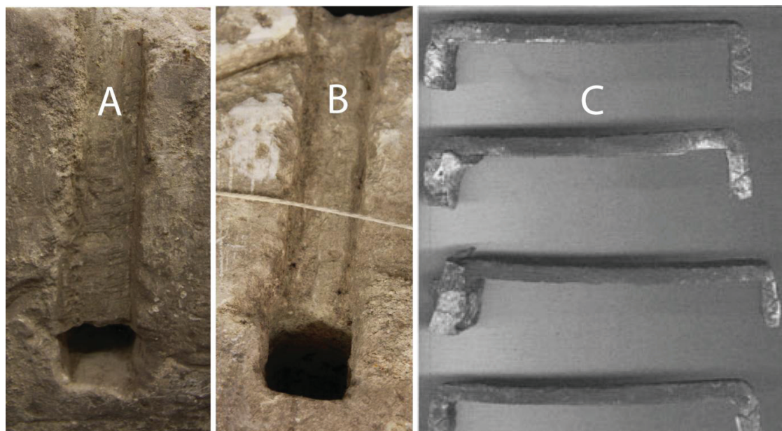
Fig. 39 : Détails des négatifs des agrafes des lots 631 (A) et 632 (B) (S. Bourocher) et exemples d'agrafes utilisées au 15 e siècle à la collégiale Saint-Nizier de Lyon aux pinacles et garde-corps extérieur (C) (N. Reveyron).
