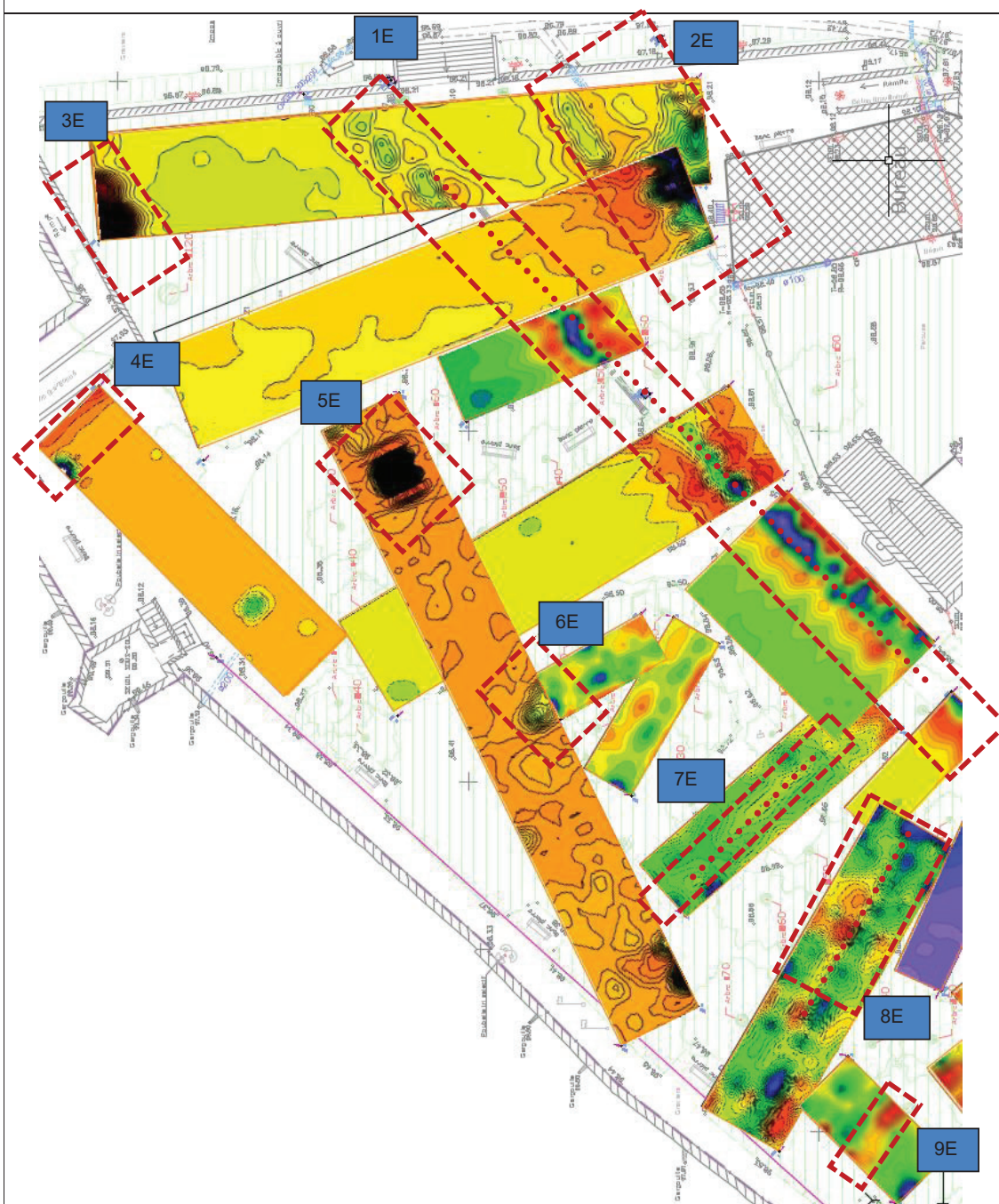
Figure 16 : mapping de la partie nord du site par méthode électromagnétique à induction
